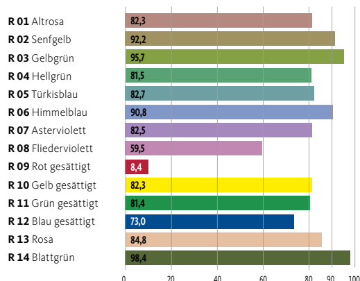
Oktalite Standard LED 3000 K R_a 83 ( 8 Testfarben) R_e 78 (14 Testfarben)
