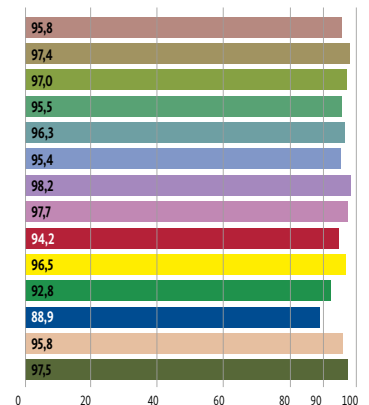
Oktalite BRILLIANT COLOUR R_a 97 ( 8 Testfarben) R_e 96 (14 Testfarben)
